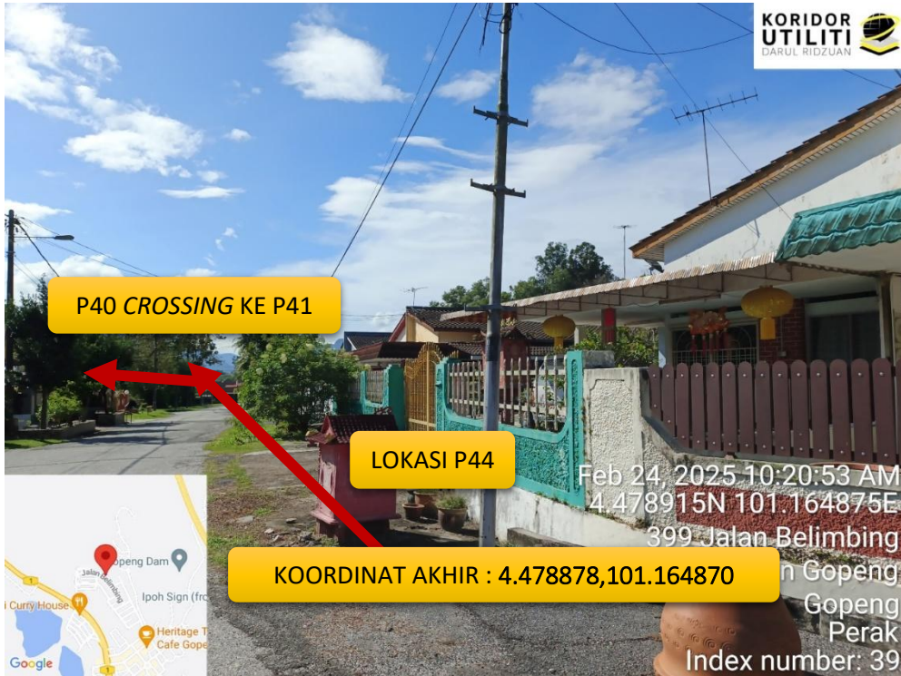
PEMASANGAN TIANG MENGIKUTI JAJARAN TIANG TNB SEDIA ADA
