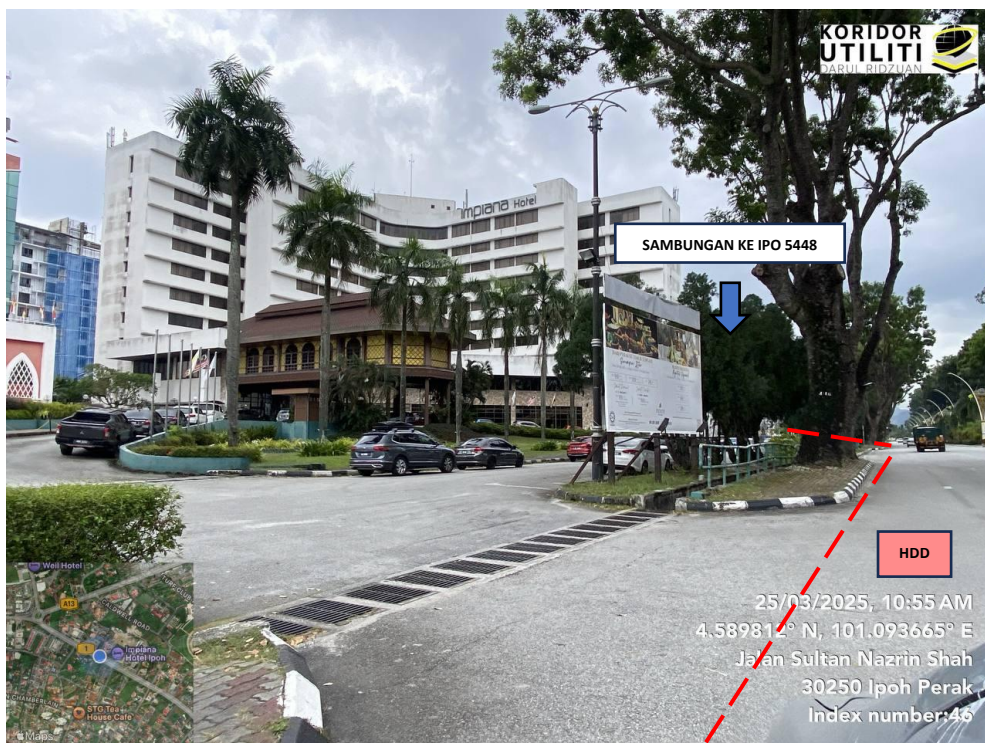
LOKASI KOORDINAT AKHIR HDD DI JALAN SULTAN IDRIS SHAH (Sambungan akan dibuat daripada PPU Hospital Bainun ke IPO 5448)
