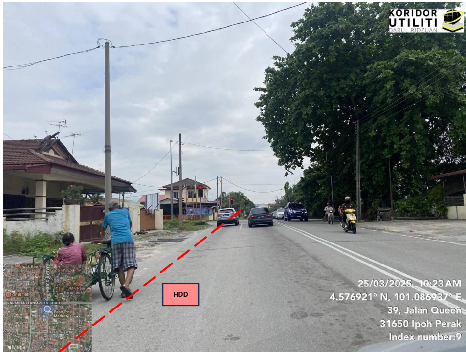
JAJARAN HDD DI JALAN QUEEN (Sambungan akan dibuat daripada PPU Pinji Lane)
