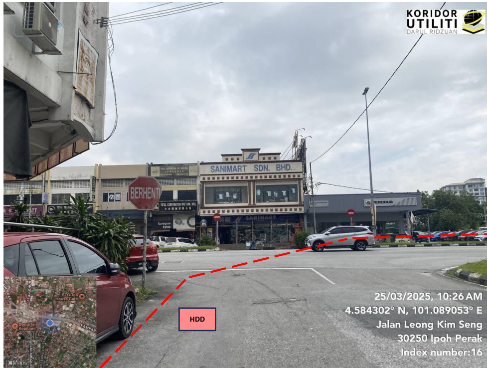
JAJARAN HDD DI JALAN LEONG KIM SENG – JALAN RAJA PERMAISURI BAINUN (Sambungan akan dibuat daripada PPU Pinji Lane)
