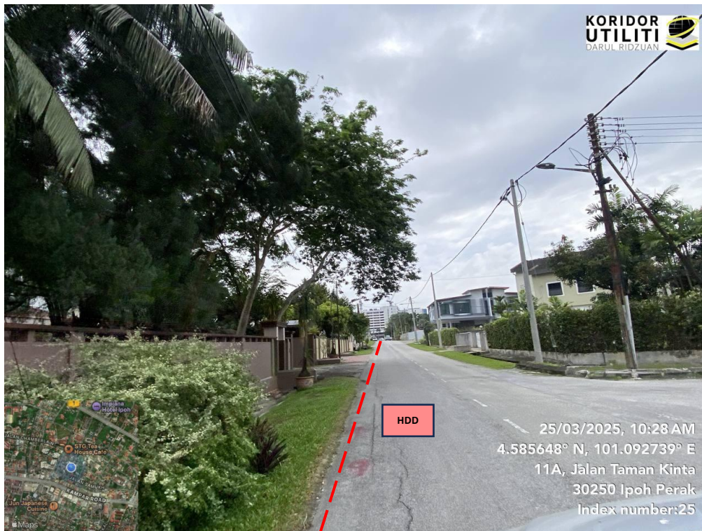
AJARAN HDD DI JALAN SAMUKH – JALAN TAMAN KINTA (Sambungan akan dibuat daripada PPU Pinji Lane ke IPO 5448)
