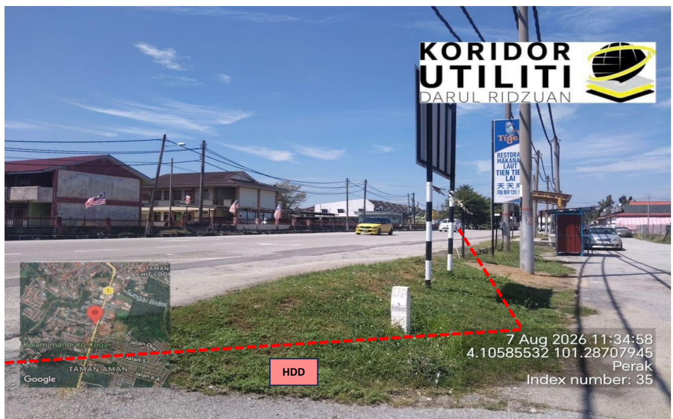
LOKASI KERJA-KERJA KOREKAN HDD DI LORONG CEGAR 2
