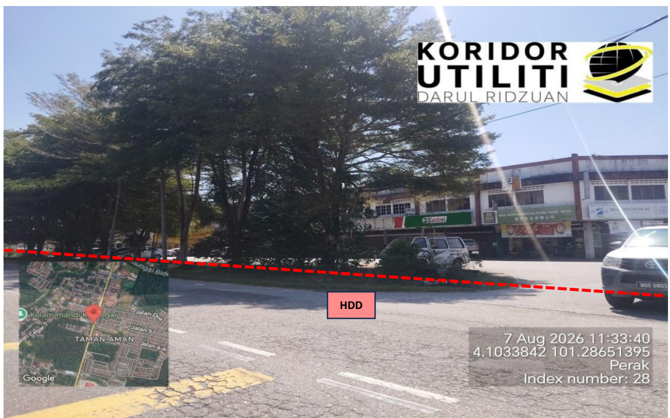
LOKASI KERJA-KERJA KOREKAN HDD DI JALAN TAMAN PUN CHUN
