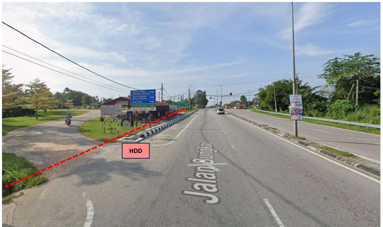
LOKASI KERJA-KERJA KOREKAN HDD DI JALAN MASUK KLINIK KESIHATAN SUNGKAI
