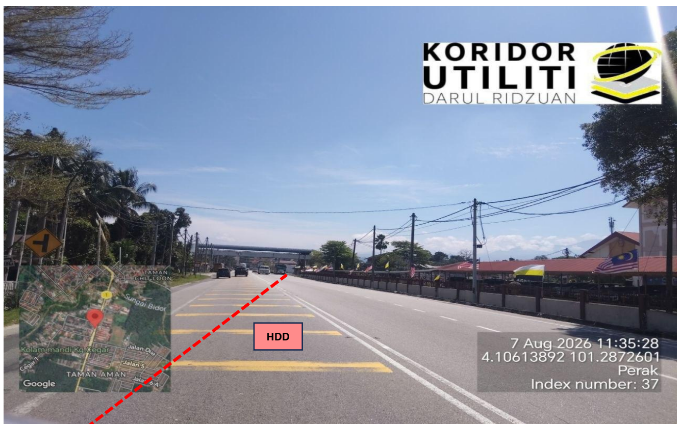
LOKASI KERJA-KERJA KOREKAN HDD CROSSING DI JALAN SUNGKAI (FT 01)
