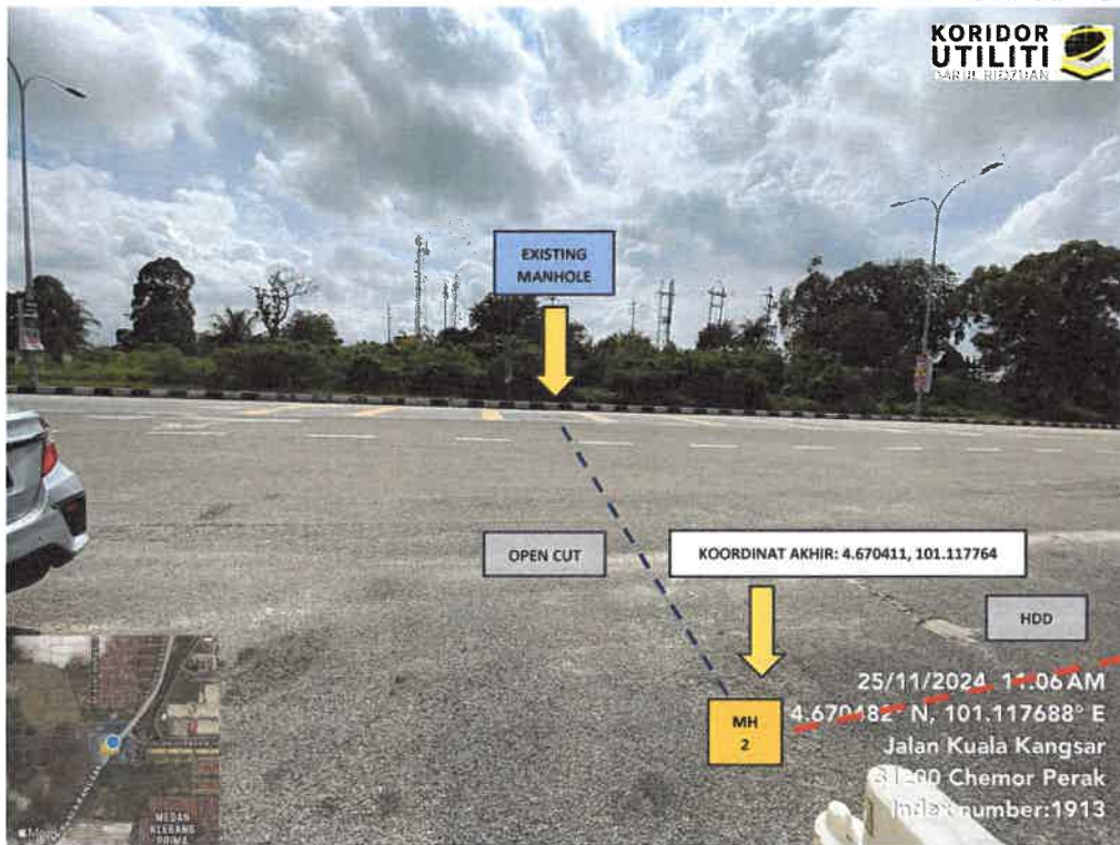
LOKASI MANHOLE CADANGAN 2 DAN MANHOLE SEDIA ADA DI JALAN KUALA KANGSAR (BERHAMPIRAN STESEN MINYAK BHP)
