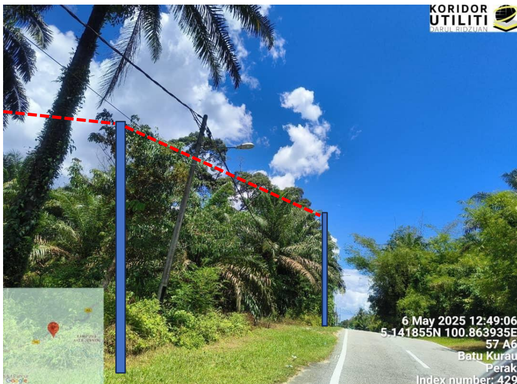
CADANGAN PENANAMAN TIANG MENGIKUT JAJARAN TIANG TNB
