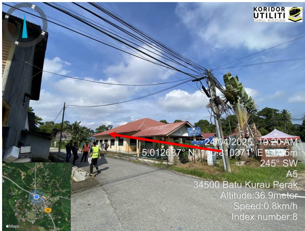
CADANGAN PENANAMAN TIANG DI JALAN KLINIK BIDAN
