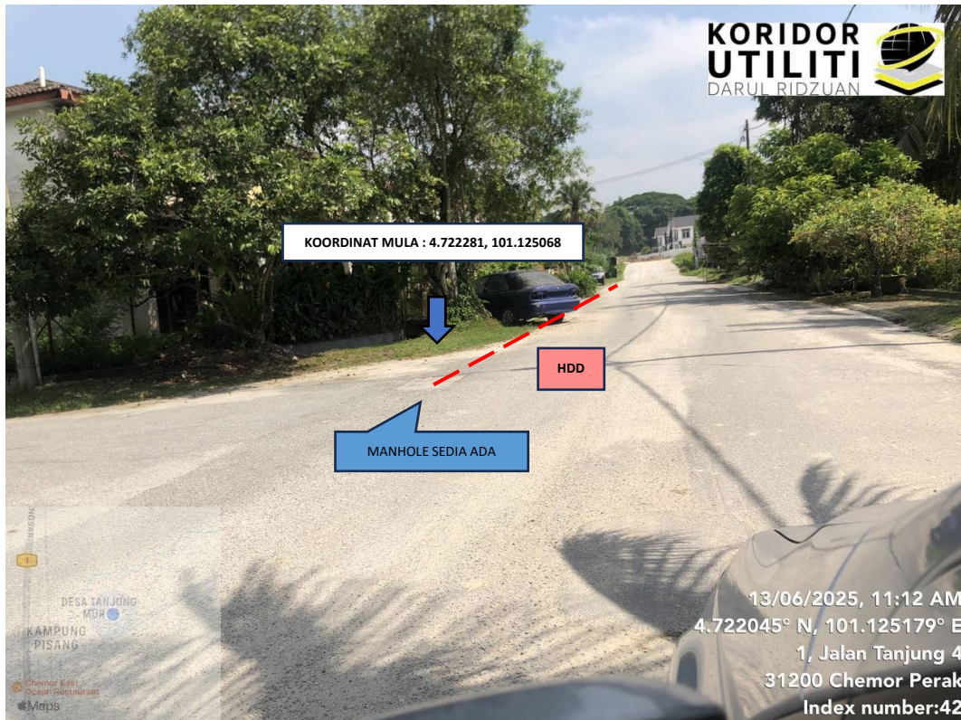
LOKASI KOORDINAT MULA KOREKAN TERBUKA DI JALAN TANJUNG 1 (Sambungan akan dibuat dari Manhole Sedia Ada ke Manhole Cadangan)
