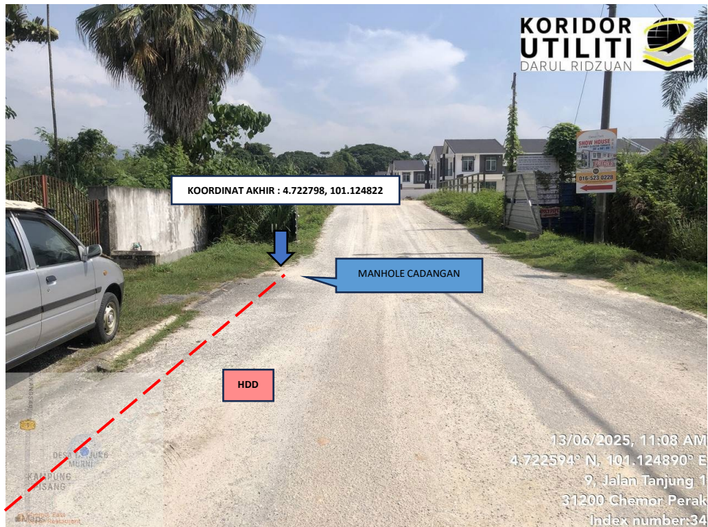
LOKASI KOORDINAT AKHIR KOREKAN TERBUKA DI JALAN TANJUNG 1 (Sambungan akan dibuat dari Manhole Sedia Ada ke Manhole Cadangan)
