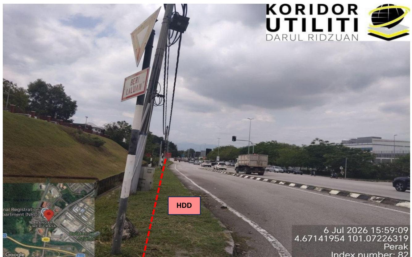
LOKASI KERJA-KERJA KOREKAN HDD DI JALAN JELAPANG - CHEMOR (A1)
