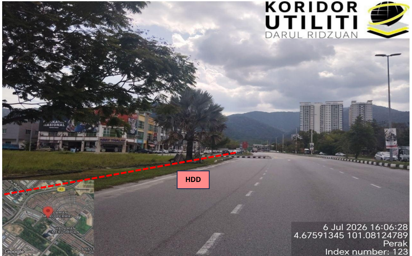
LOKASI KERJA-KERJA KOREKAN HDD DI JALAN MERU @JALAN LEBUH MERU (A268)
