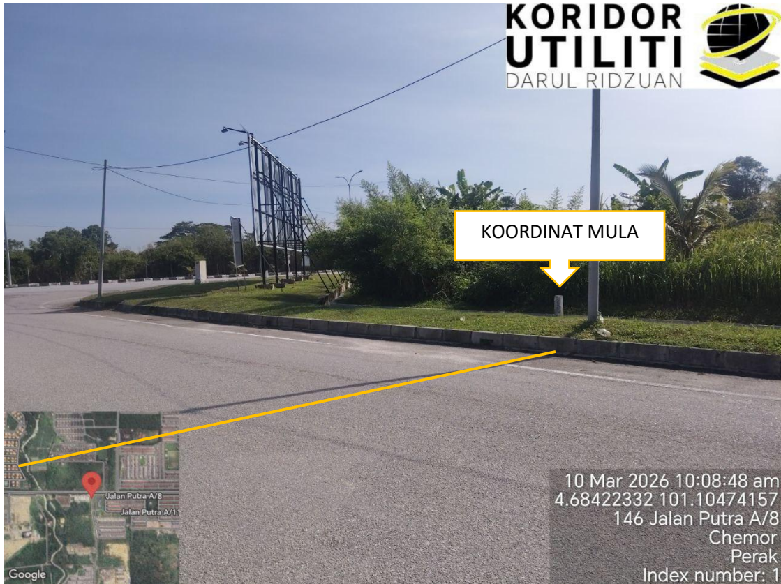
KOREKAN TERBUKA DI JALAN BERTURAP (CW) SEPANJANG 9 METER
