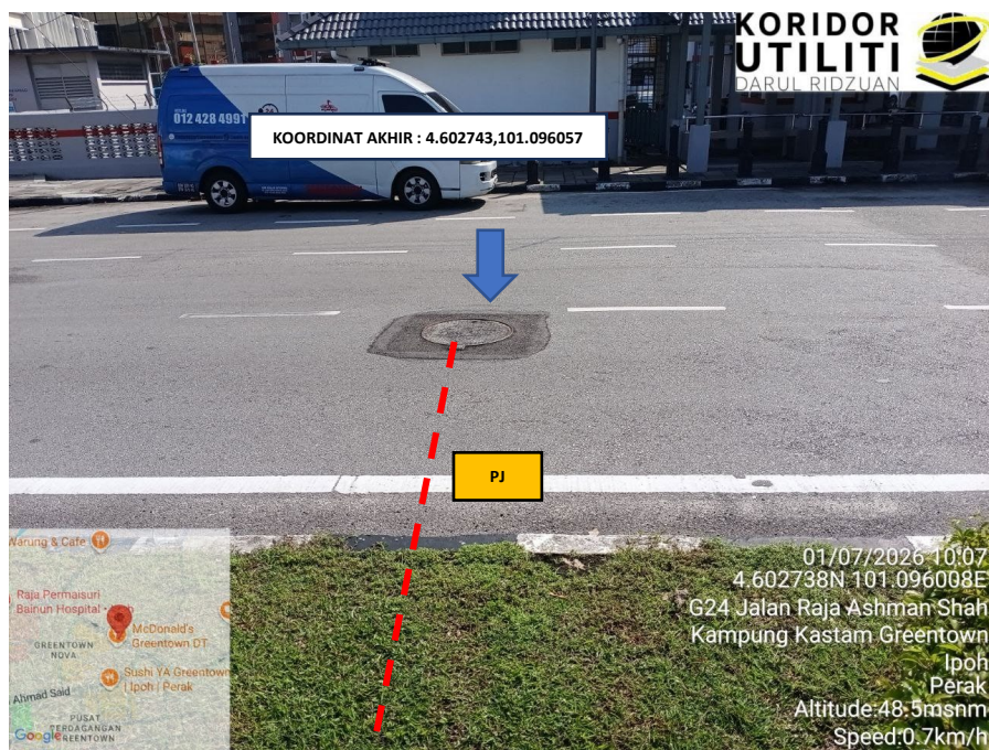
LOKASI KOORDINAT AKHIR PIPE JACKING DI JALAN RAJA ASHMAN SHAH
