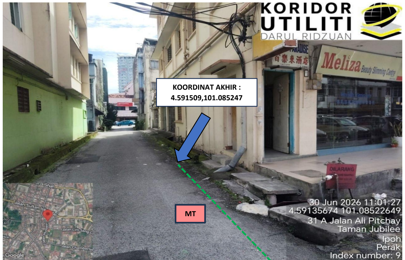
LOKASI KOORDINAT AKHIR KERJA KOREKAN TERBUKA MICRO TRENCHING DI JALAN ALI PITCHAY ( LORONG TENGAH )
